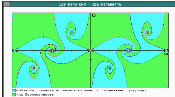
Рис. 3.1. Фазовый портрет без дополнительных седел
