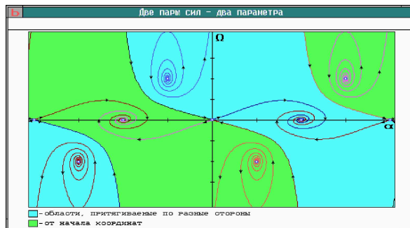
Рис. 3.2. Фазовый портрет без дополнительных седел
